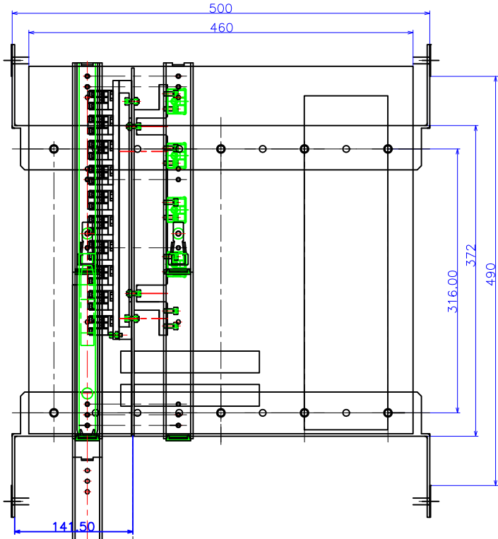
インターロック盤 マウントラック組立図 2015年5月31日 東谷
